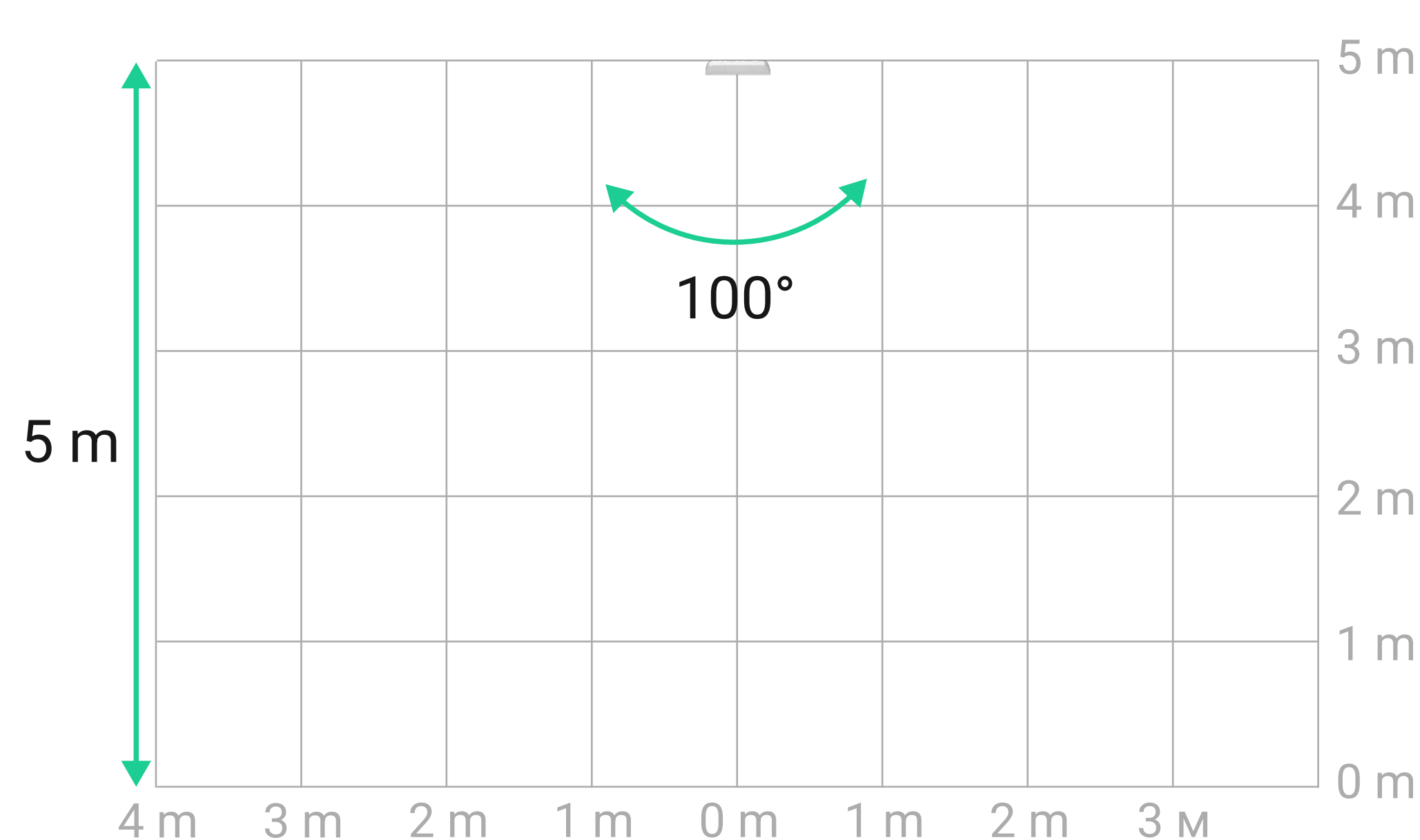
Vue horizontale
